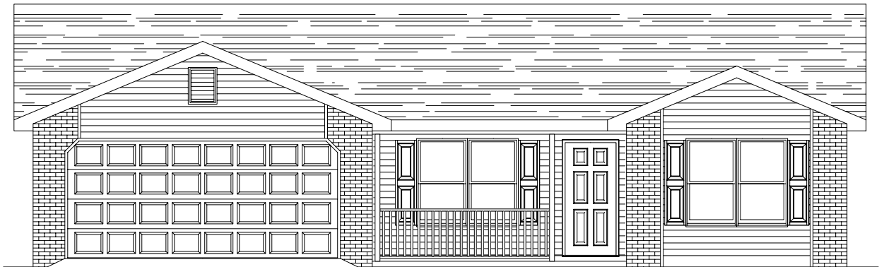
ELEVATION "C"
